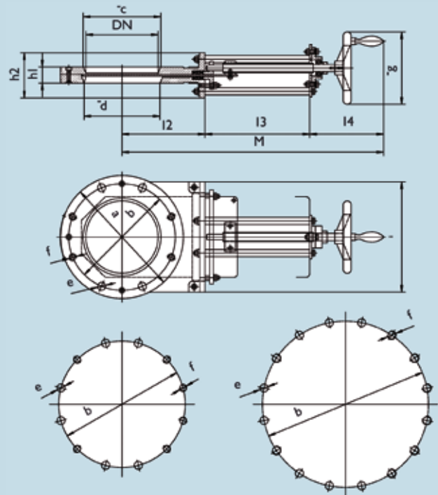
Die Abbildung zeigt einen Flachschieber mit Handrad und Gewindespindel.
